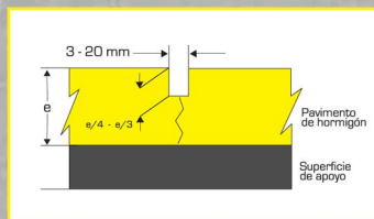
Junta de contracción
